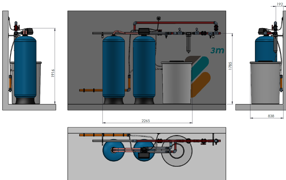
Dimenzije i izgled omekšivača Omekšivač aqua3M D200
